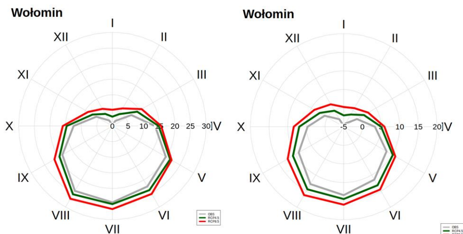
Rysunek 2. Przebieg roczny temperatury powietrza minimalnej i maksymalnej dobowej [°C] w Wołominie w okresie 2071-2090, symulowanego w dwóch eksperymentach RCP4.5 (linia zielona) i RCP8.5 (linia czerwona), linia szara oznacza wartości referencyjne (obserwowane) z okresu 1971-2017
